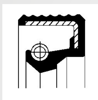
Figura 2: anello di tenuta 12010784B nuovo design
