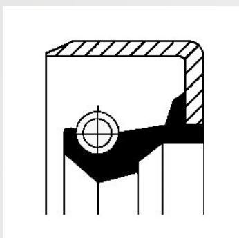
Figura 1: anello di tenuta 01002369B design precedente
